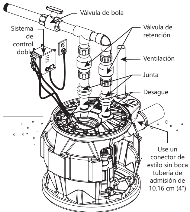
Figura 2. Instalación típica (se muestra la serie Pro680)
