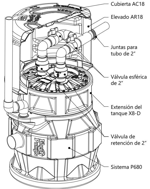
Figura 1. P680 Instalación típica para exteriores
